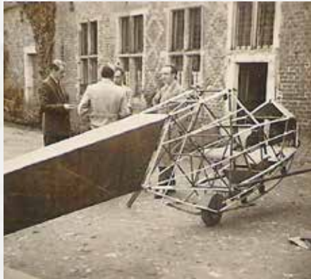
↑Bild 5: Besprechung einiger Fliegerkameraden beim Bau des Doppelsitzers
